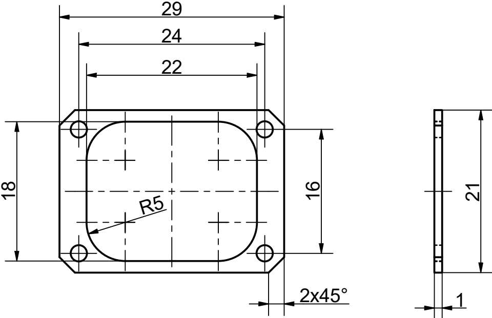
Pos. 2: Top-Plate
