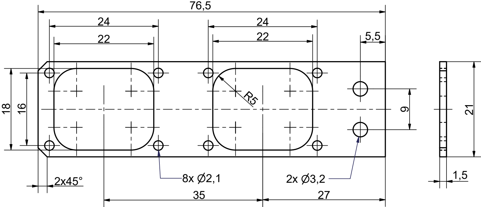
Pos. 1: Ground-Plate
